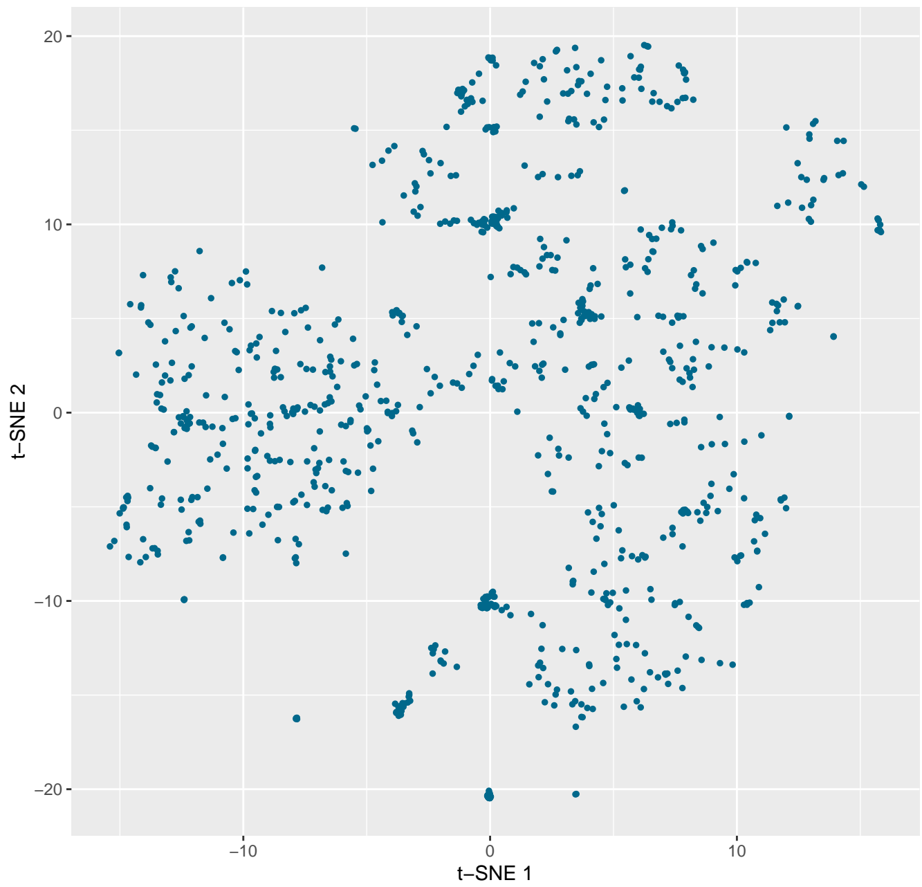
t-SNE
