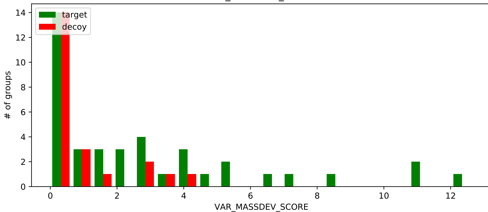
VAR_MASSDEV_SCORE
