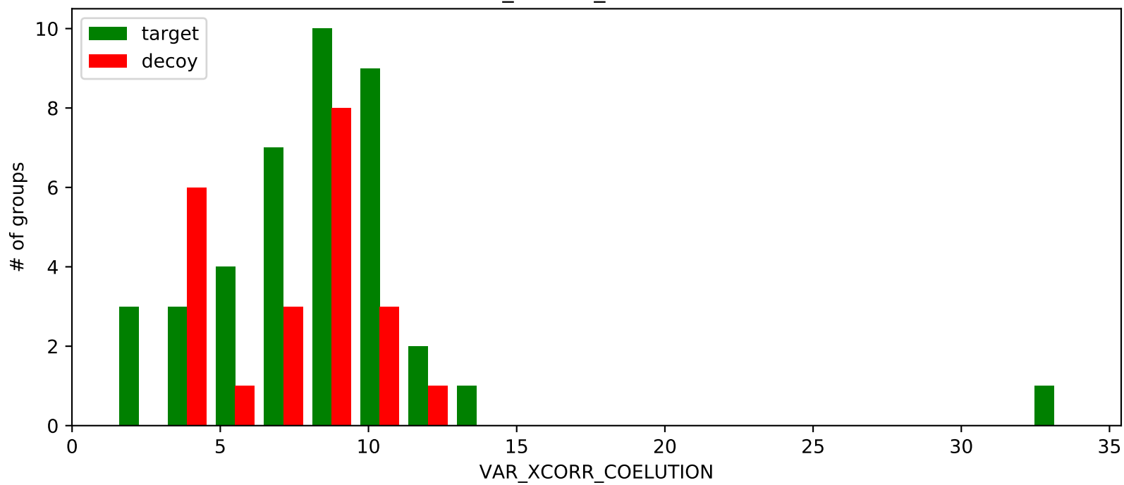
VAR_XCORR_COELUTION
