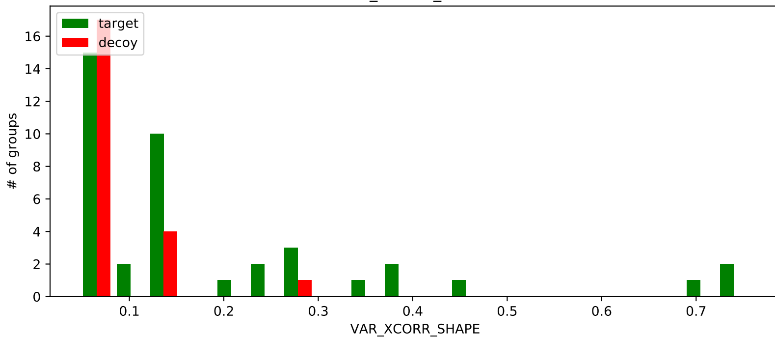
VAR_XCORR_SHAPE
