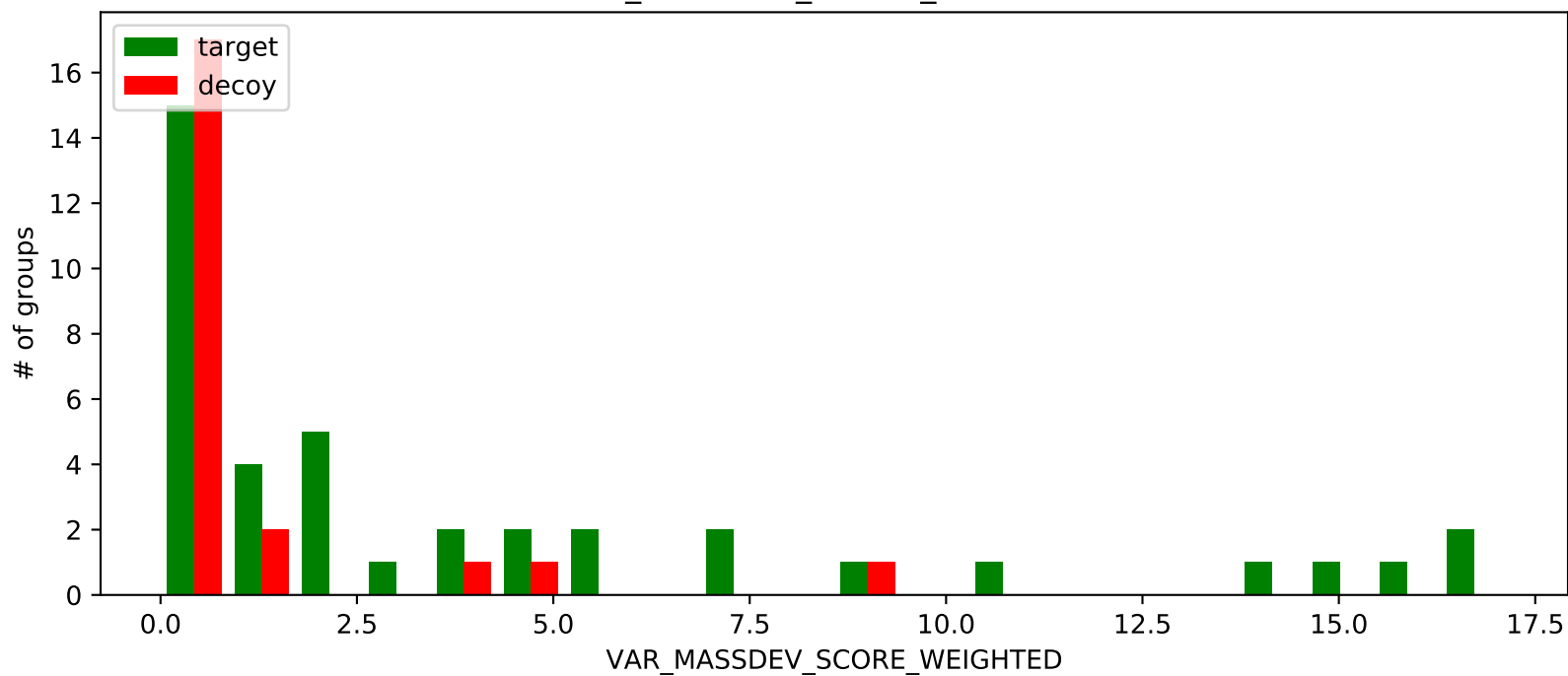
VAR_MASSDEV_SCORE_WEIGHTED
