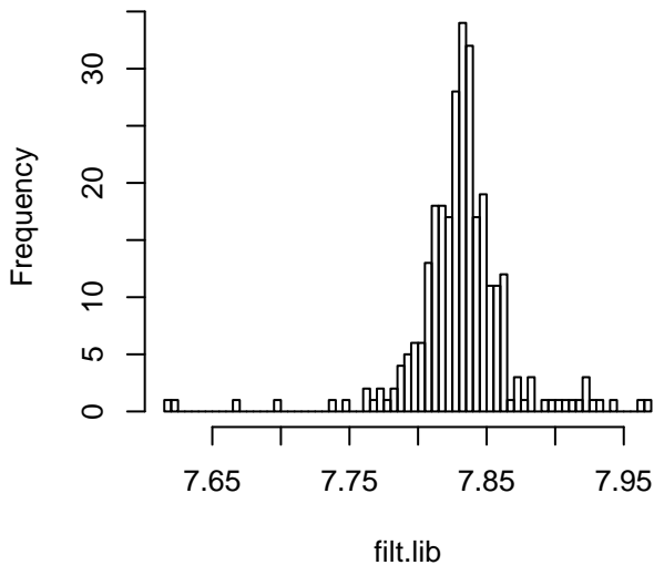
FiltData Log(LibSize)
