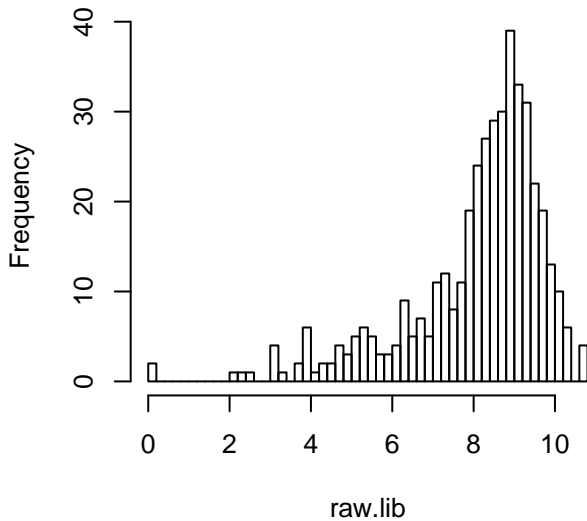
ExpData Log(LibSize)
